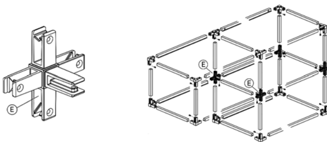
5-weg hoekverbinder Float type 861AZ5
