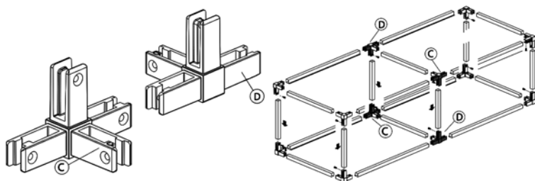
4-weg hoekverbinder Float type 861AZ3/4
